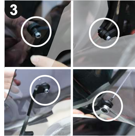
Camı ayaklara konumlandırıp paket içerisinden çıkan civata, plastik pul, plastik conta ve somunları 3 alyan ve 8 anahtar yardımıyla sabitleyiniz. (Position the glass onto the feet and secure it using the bolt, plastic washer, plastic gasket, and nut from the package, with the help of a 3 Allen wrench and an 8 wrench.)
